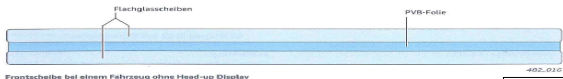
Frontscheibe bei einem Fahrzeug ohne Head-up Display
