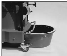
Staubwanne zurückschieben.
