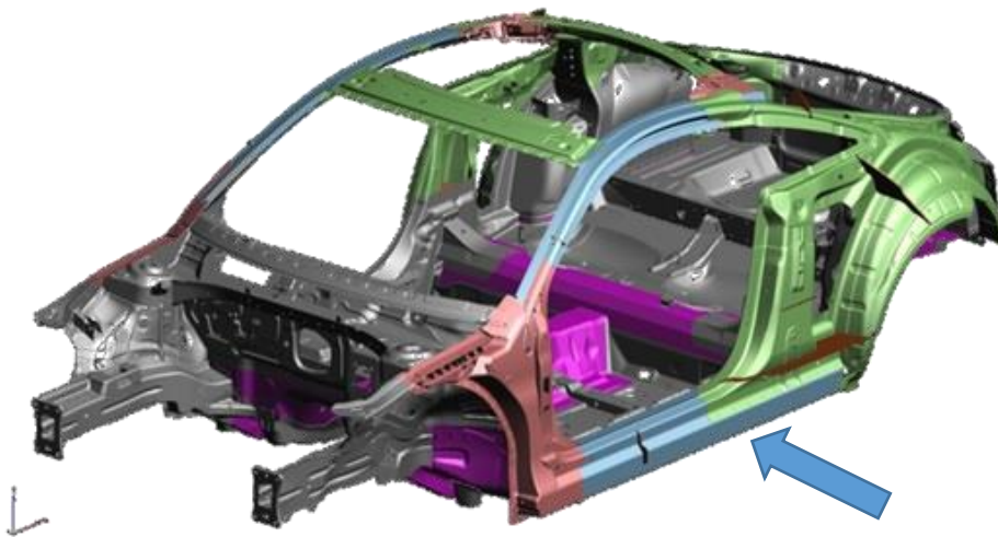
Schnitt durch AL und ST gleichzeitig
