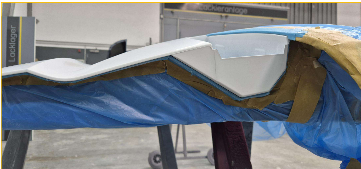
Bild 10: Werkstattbild Heckklappe Neuteil seitlich/innen abgedeckt zur Außenlackierung im Grundfarbton „Rot“
