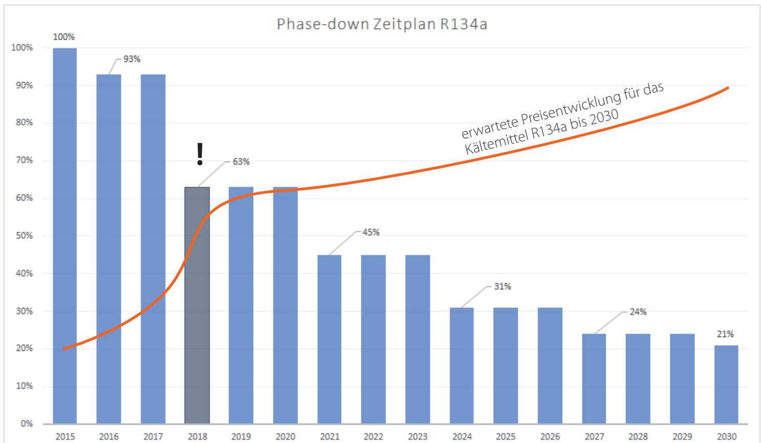
Abbildung: Phase-Down Zeitplan mit der wahrscheinlichen Preisentwicklung für das Kältemittel R134a (Quelle: European Partnership for Energy and the Environment)
